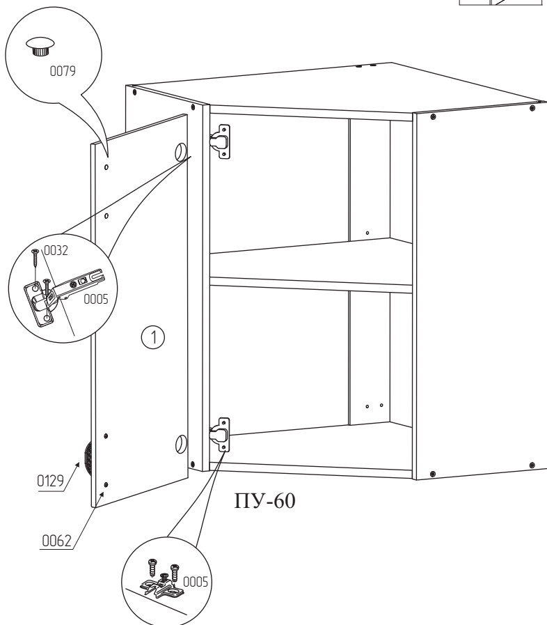
вариант навески фасада слева
